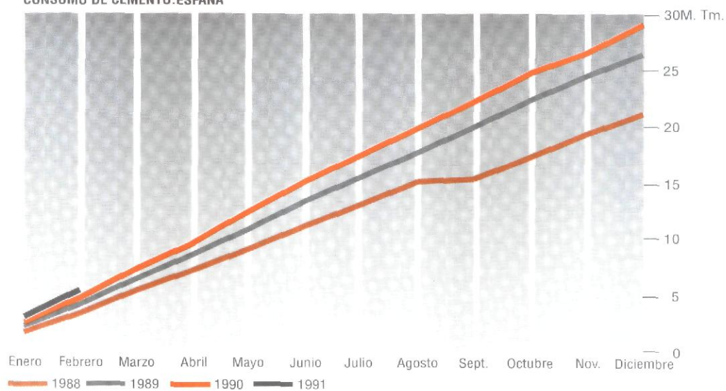
CONSUMO DE CEMENTO. ESPAÑA
